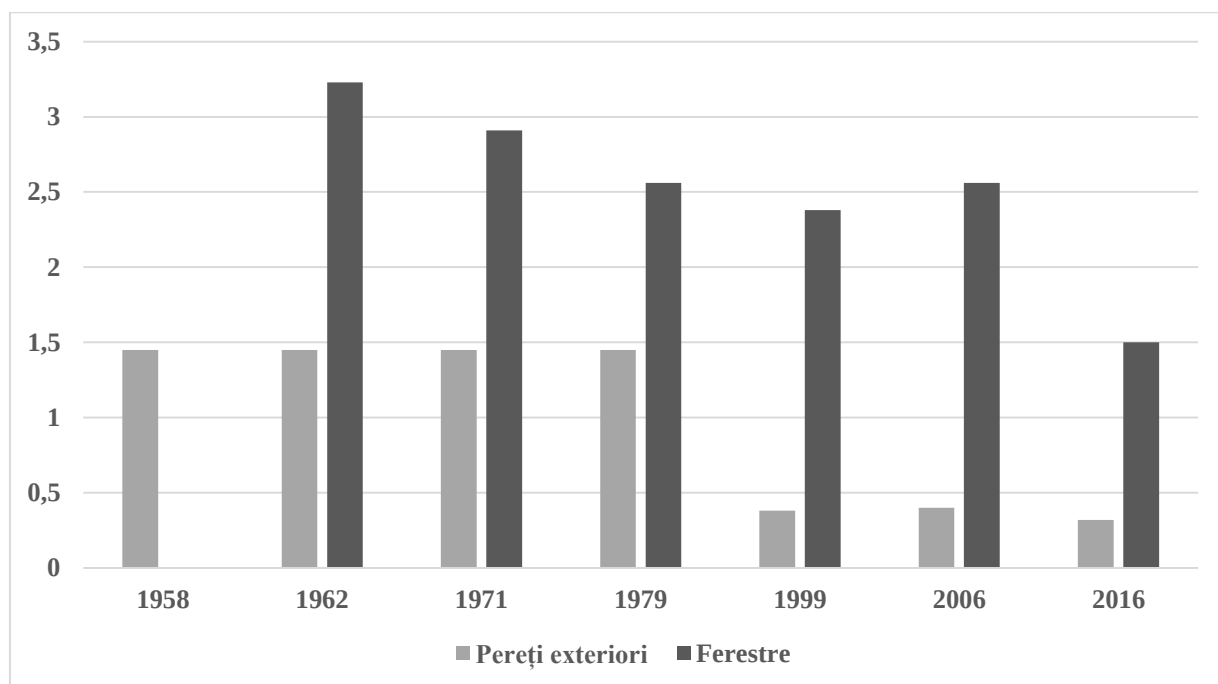
Figura 2. Evoluția cerințelor privind coeficientul maxim de transfer de căldură (valoarea U) pentru unele elemente ale anvelopei clădirii
